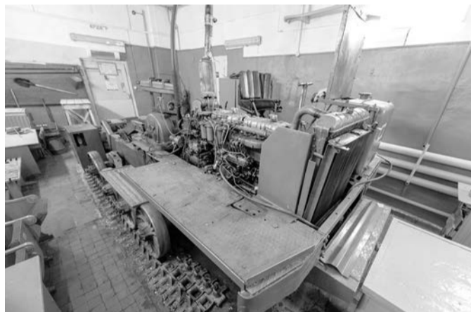
На этом «стационарном» тракторе студенты обучаются первым навыкам управления лесозаготовительной техникой
